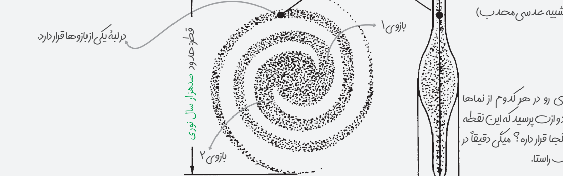
شکل ۱-۵: طرح شماتیک یک کهکشان مارپیچ مانند کهکشان راه شیری
