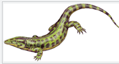
شکل ۱-۸- هیالونوموس نخستین خزنده یافت شده در ابتدای کربونیفر با طول حدود ۱۲ سانتی متر
