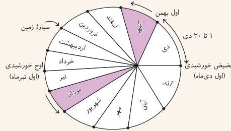
نمایش قانون دوم کپلر
