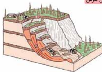
مدل لغزش
